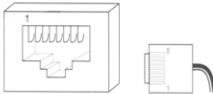
图2.5 SD732设备的网络维护接口形状
