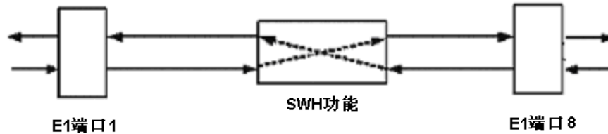
图 1 SD732 的交叉功能示意图
