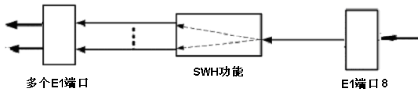
图 2 SD732 的交叉功能示意图
