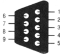
图2.4 SD732设备的操作维护接口形状以及引脚顺序
